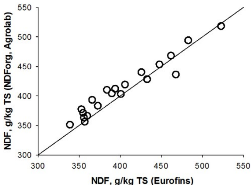
Figur 1. Sammenligning af NDF koncentration i kløvergræsensilage bestemt ved Eurofins og Agrolab. Ved begge laboratorier er anvendt askekorrektion af NDF-resten. Hvert punkt repræsenterer én ensilage (n = 20; r = 0,97).
